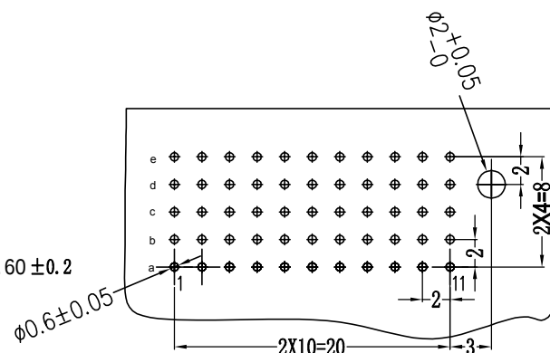
固定PCB板尺寸 (公差 \pm 0.05 )
