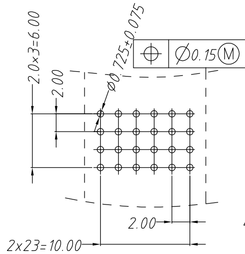
PCB LAYOUT (公差 ± 0.05)
